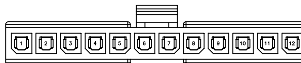
12PIN
