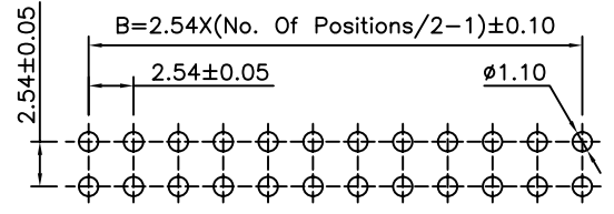
P.C.B. Layout
