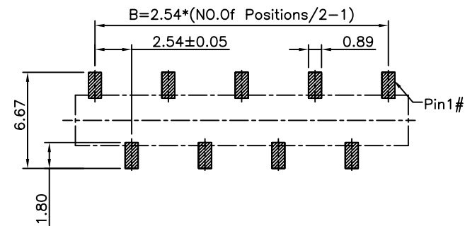
P.C.B. Layout(B2 Type)
