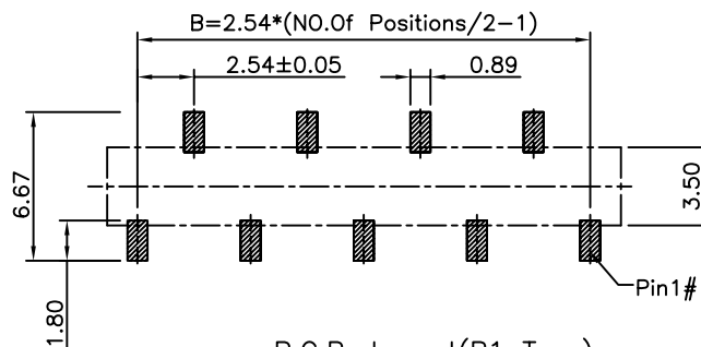
P.C.B. Layout(B1 Type)
