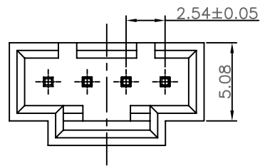
(4~18 Pin)
