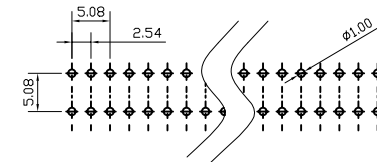
P.C.B LAYOUT
